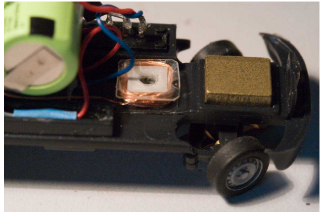
Foto 16: Een plaatsje voor de ontvangstspoel
