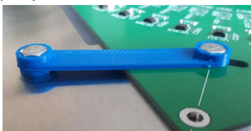
Figuur 4: Gebruik borgplaatje
