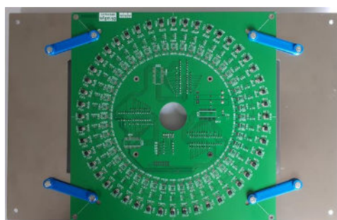
Figuur 5: Verlengplaat bevestigd aan DTS (links bovenaanzicht, rechts onderaanzicht)
