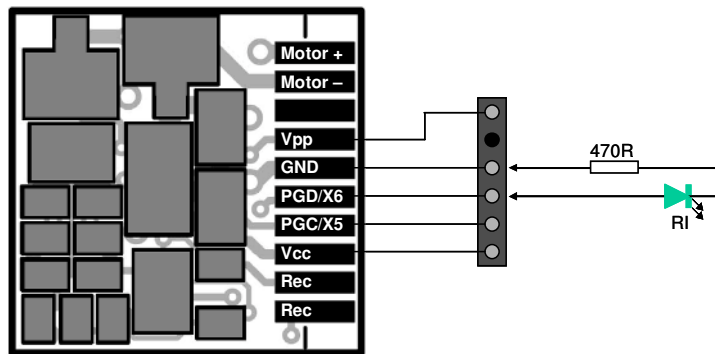
Fig 8: Aansluiten programmeerinterface
