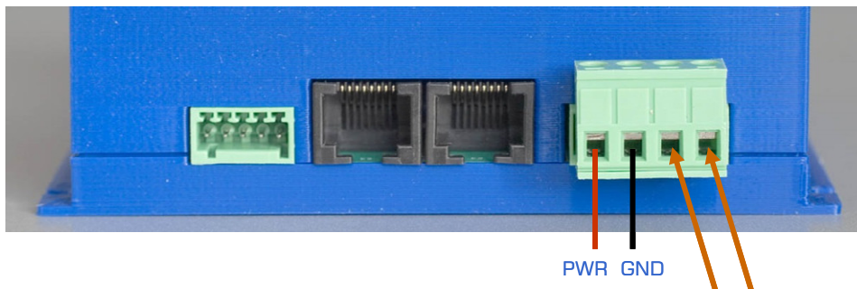
Fig. 12 : Connexion de l'alimentation au TM44 NE BRANCHEZ PAS!
