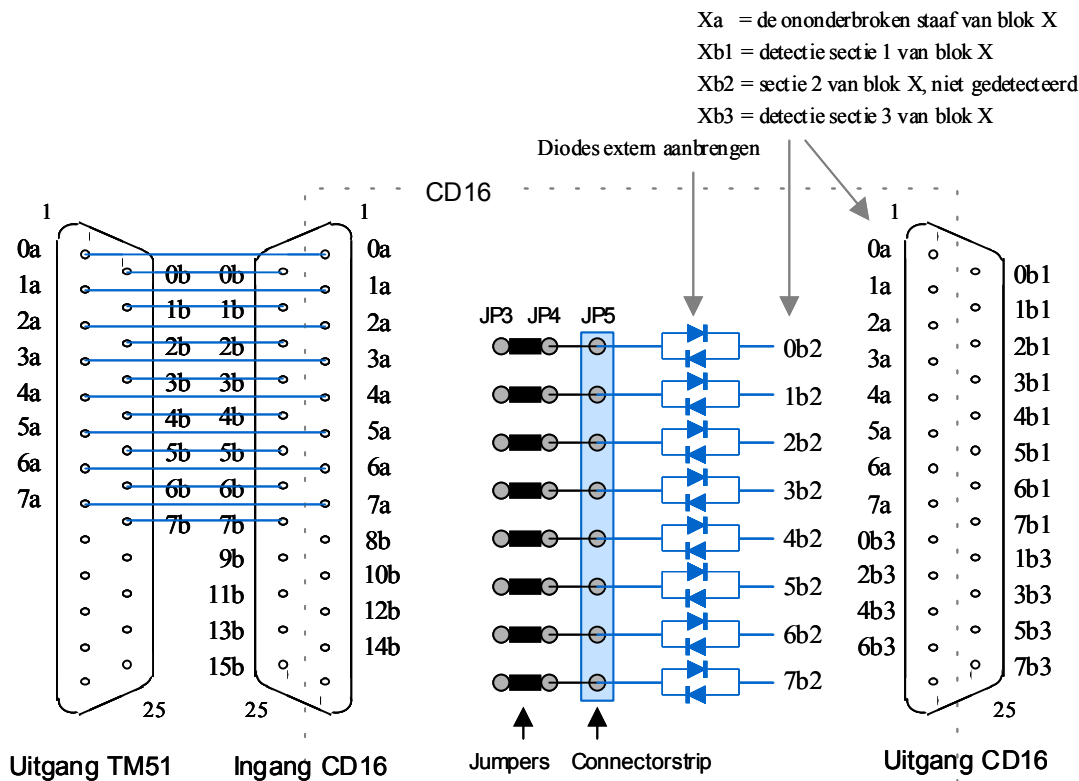
fig 10: 'Slim' aansluiten van de CD16 voor 3 secties per blok
