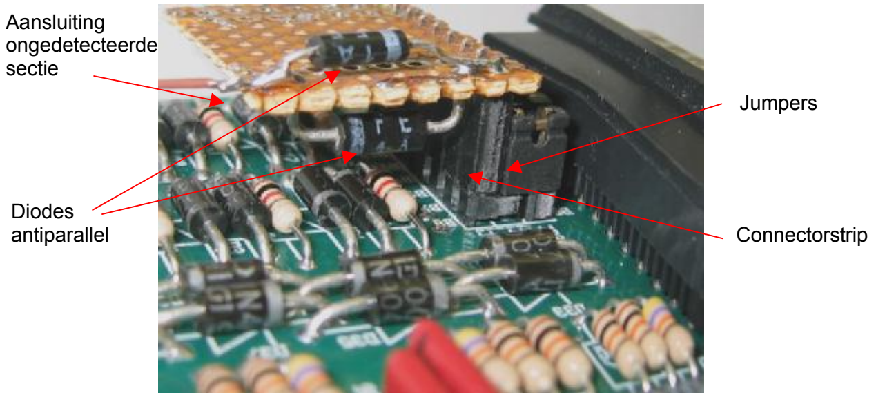
fig 11: Praktische uitvoering aansluiten ongedetecteerde secties
