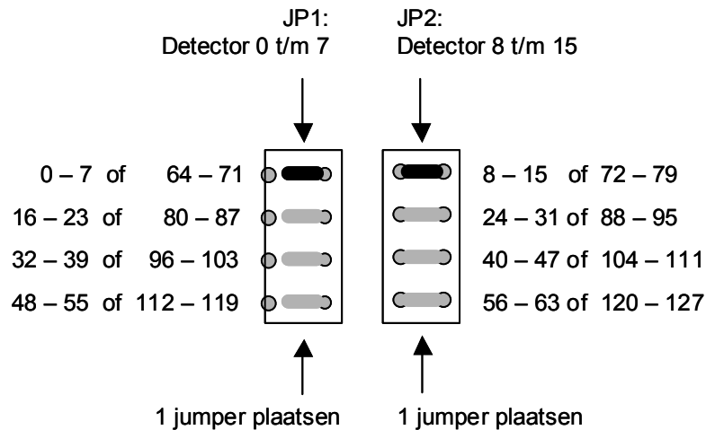
fig 13: Adres selectie van de CD16
